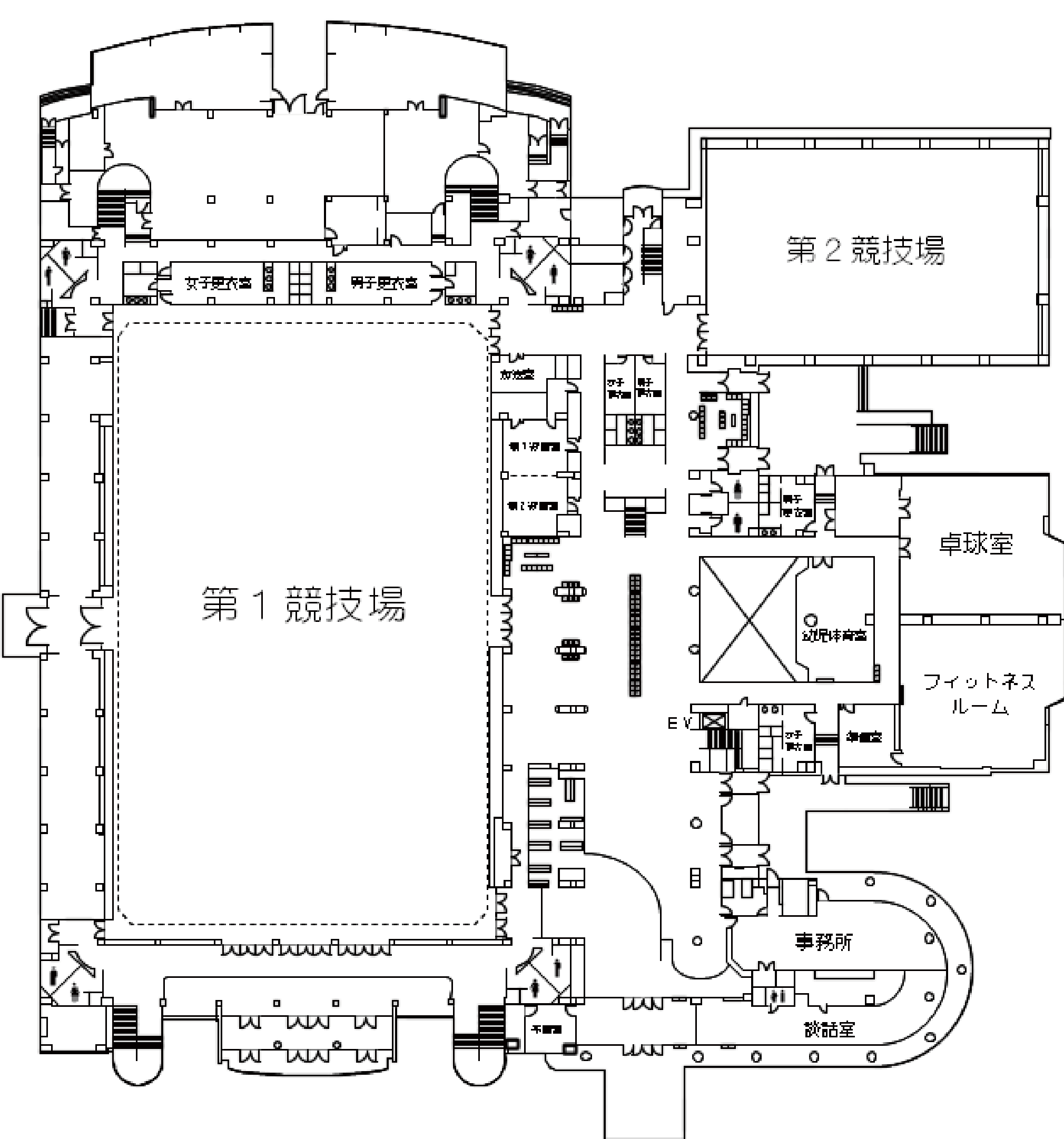
1階平面図
