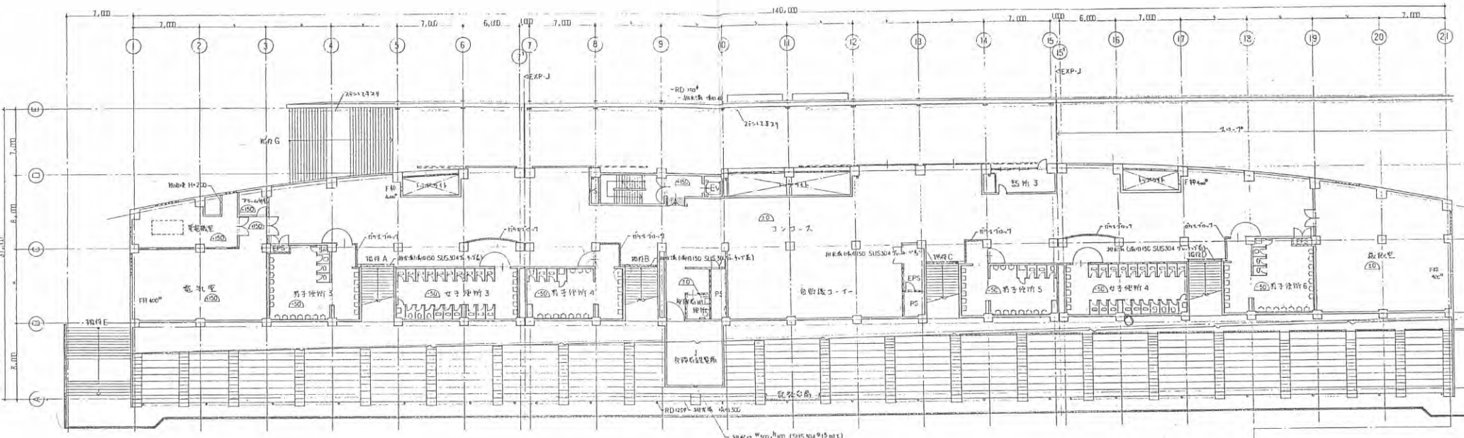
2 階平面図 1:200
