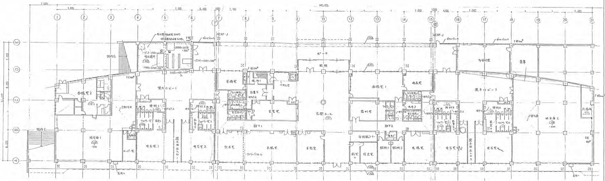
1 楼层平面图 1:200
